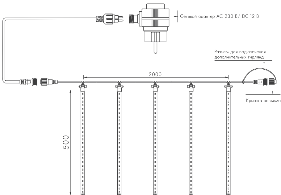
Рисунок 1. Схема подключения.
